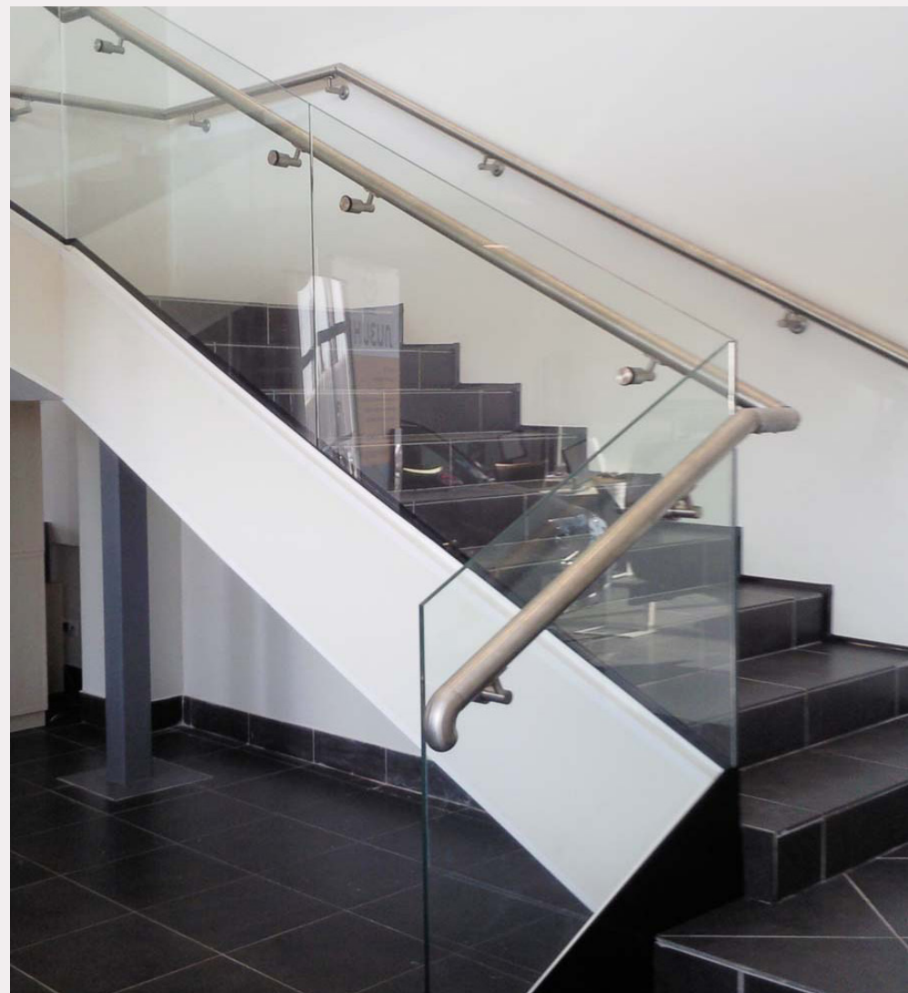
объект: салон Volkswagen материал поручня: сталь триплекс 8+8 закаленный открытое крепление стекла к маршу лестницы
